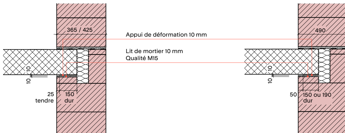
Porotherm 365 et 425 mm
